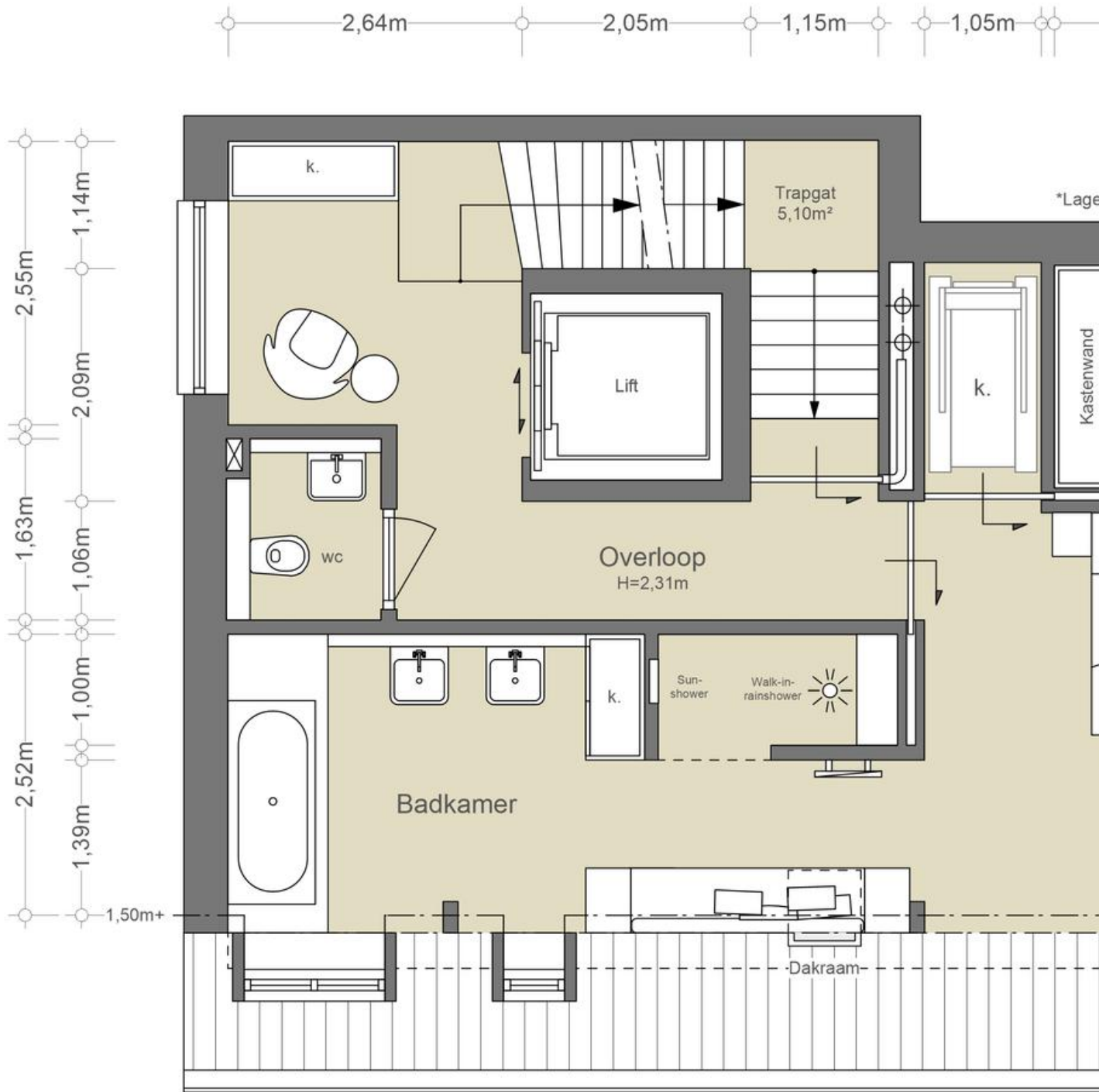
2 e VERDIEPING
